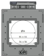
Masszeichnung-2
