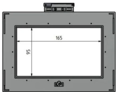
Masszeichnung-2
