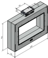
Masszeichnung-1
