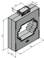
Masszeichnung-1
