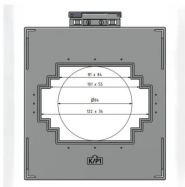
Masszeichnung-2
