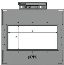
Masszeichnung-2
